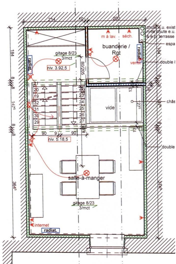
Deuxième étage
